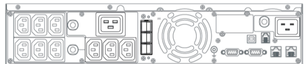
Back (ELITE PRO 2200ELCDRTXL2U)
