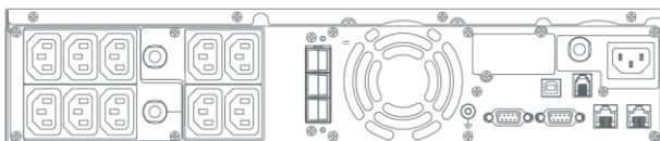
Back (ELITE PRO 1000/1500ELCDRTXL2U)
